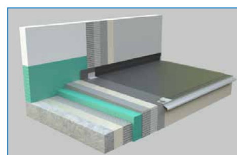
10. NANIESŤ DRUHÚ VRSTVU HYDROIZOLÁCIE EXCEL MIX 2K
