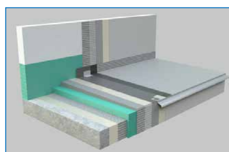
11. NANIESŤ LEPIDLO NA DLAŽBU TS FLEX, TS FLEX PLUS ALEBO TS EXCELQUICK
