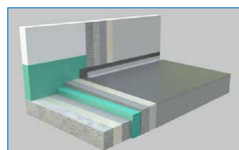
7. DO ROHOV A KÚTOV VLOŽIŤ TESNIACI PÁS 2K
