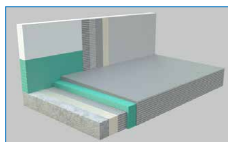
5. VYTVORIŤ SPÁDOVÚ VRSTVU VÝROBKOM VYROVNÁVAJÚCA STIERKA
