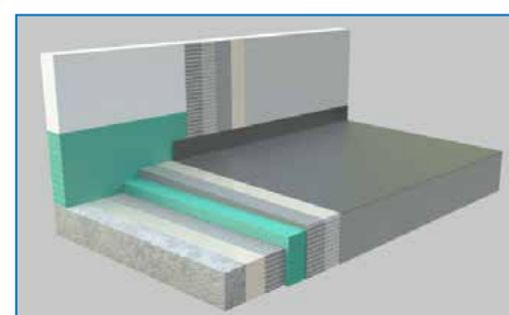
6. NANIESŤ PRVÚ VRSTVU HYDROIZOLÁCIE EXCEL MIX 2K NA SOKEL A PLOCHU
