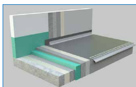
8. OSADIŤ BALKÓNOVÝ PROFIL
