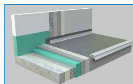
9. BALKÓNOVÝ PROFIL PRELEPIŤ SAMOLEPIACOU TESNIACOU PÁSKOU
